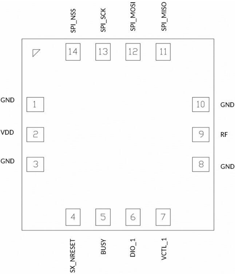
图 1.1 引脚分布图
