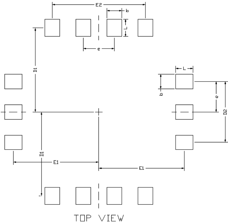
图 3.3 Footprint 尺寸
